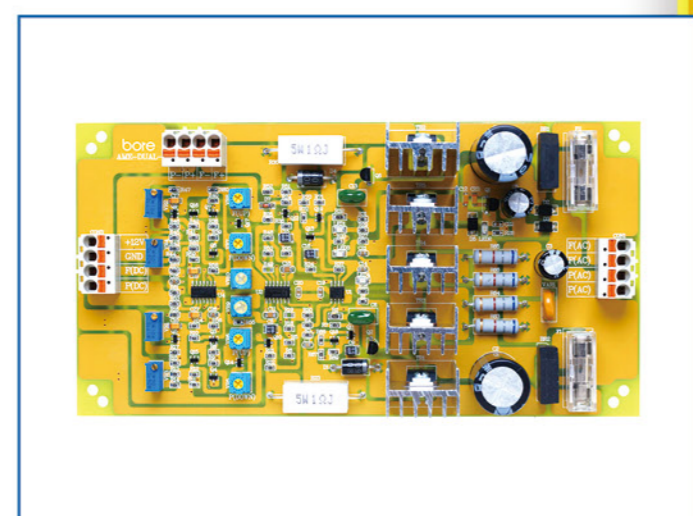
▲ 比例閥控制板 PCB 整合案例
