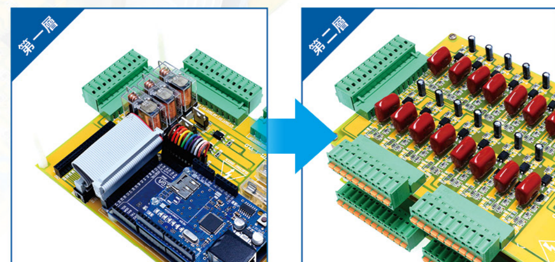
▲ 搭配 ARDUINO PCB 板，採用雙層設計，以塑膠柱做堆疊的 PCB 整合案例
