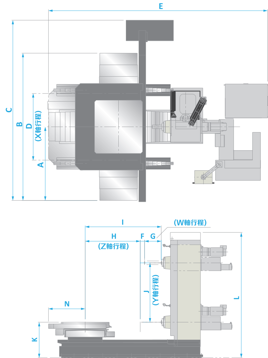
BMC-R 型 外型尺寸&加工範圍
