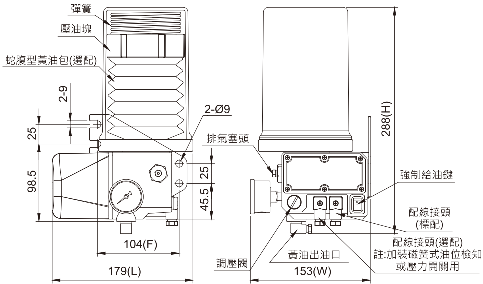
KABP-07 外型圖 (加裝磁簧式油位檢知、壓力開關，蛇腹型黃油包另購)
