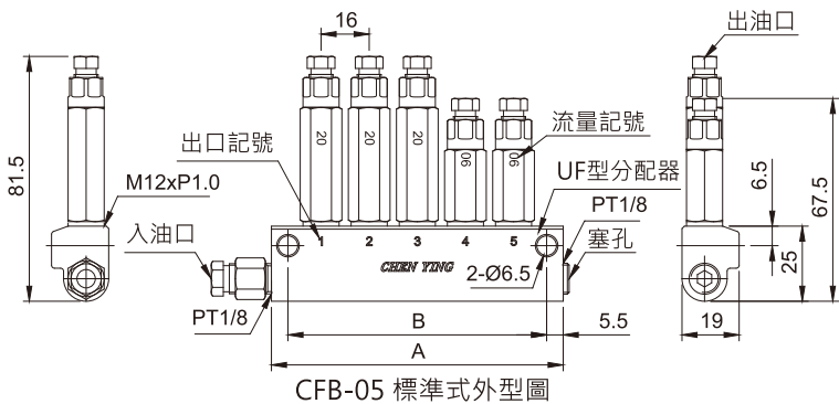
CFB-05 標準式外型圖
