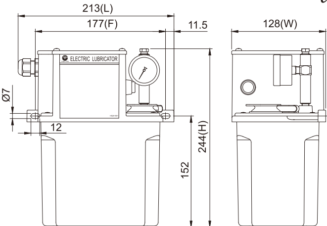
CEN03 標準品外型圖
