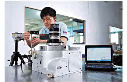
雷射(激光)測量儀 檢驗分度盤 分割精度
