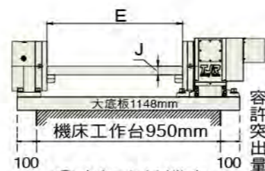
④底板大於機床工作台的示意圖
