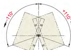
A矢視圖:傾斜軸旋轉角度
