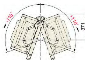
A矢視圖:傾斜軸旋轉角度
