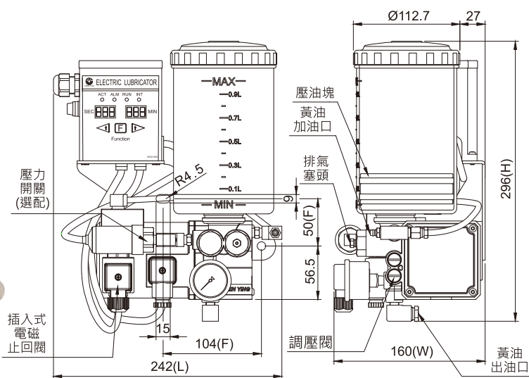
KGNB-35 (電動脫壓)外型圖 (加裝壓力開關)
