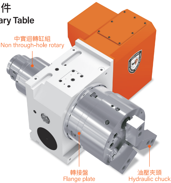
數控旋轉工作台與夾頭選配表 / Rotary Table and Compatible Chuck
