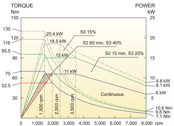
FANUC 20HP (OPT) Model : 850 / 1050 / 1100 / 1300
