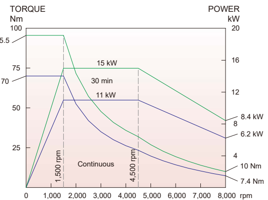
MITSUBISHI 20HP (OPT) Model : 850 / 1050 / 1100 / 1300
