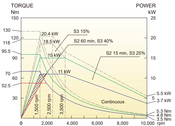
FANUC 20HP Model : 850 / 1050 / 1100 / 1300
