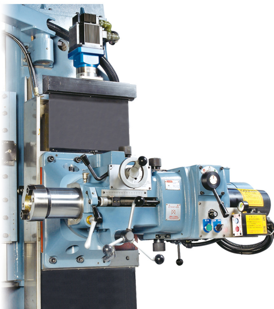
HK砲塔式主軸(主軸可伸縮)
