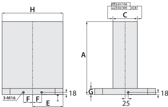
規格表 (材質: 高精密 FCD 50 石墨鑄鐵 / 鋁合金 A356)
