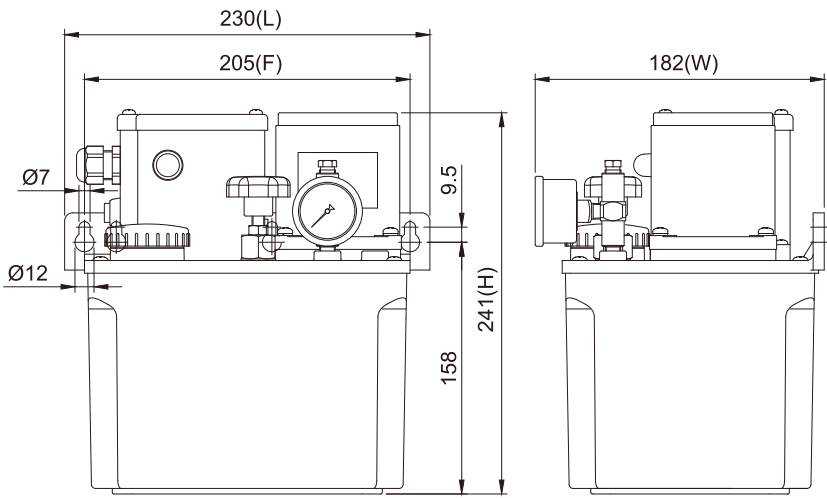
CEVB-03-25W 外型圖 (加裝強制給油鍵、指示燈)
