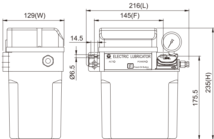
CESG03 標準品外型圖
