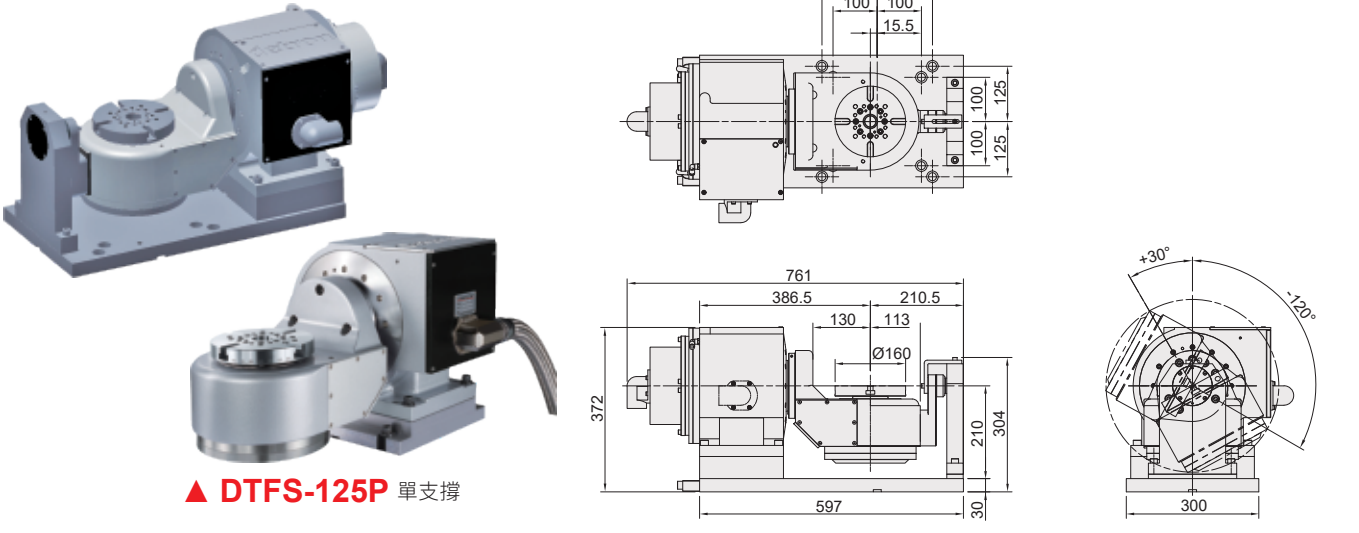
DTFE-125P 平底型
