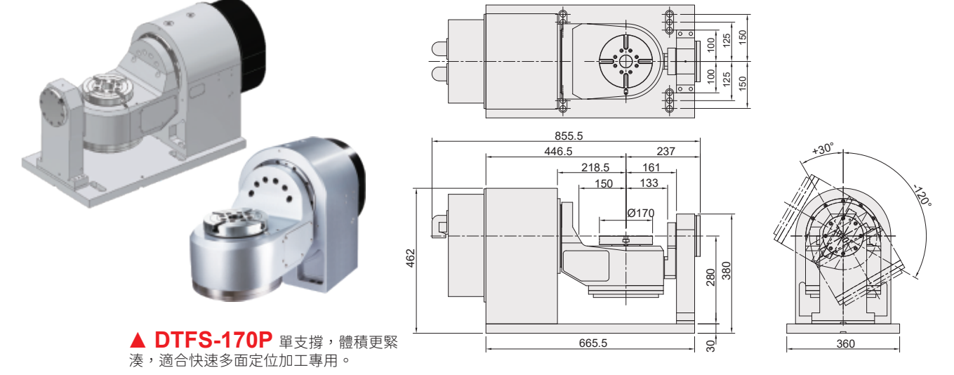
DTFE-170P 平底型
