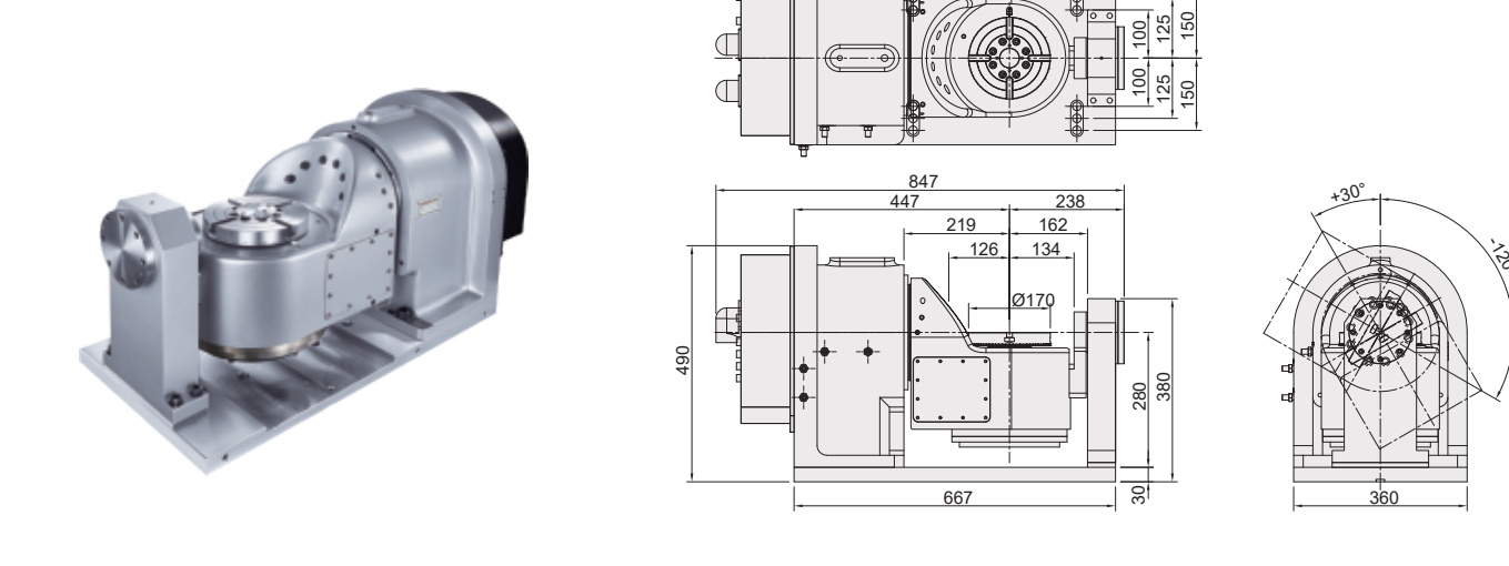
DTFE-171P
