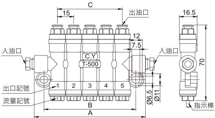
T-500 快插式外型圖
