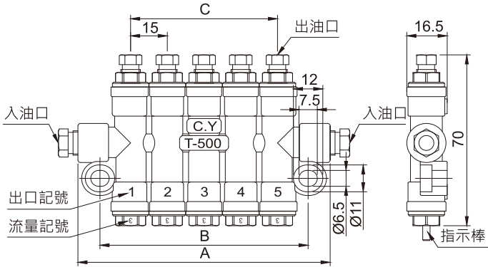
T-500 標準式外型圖
