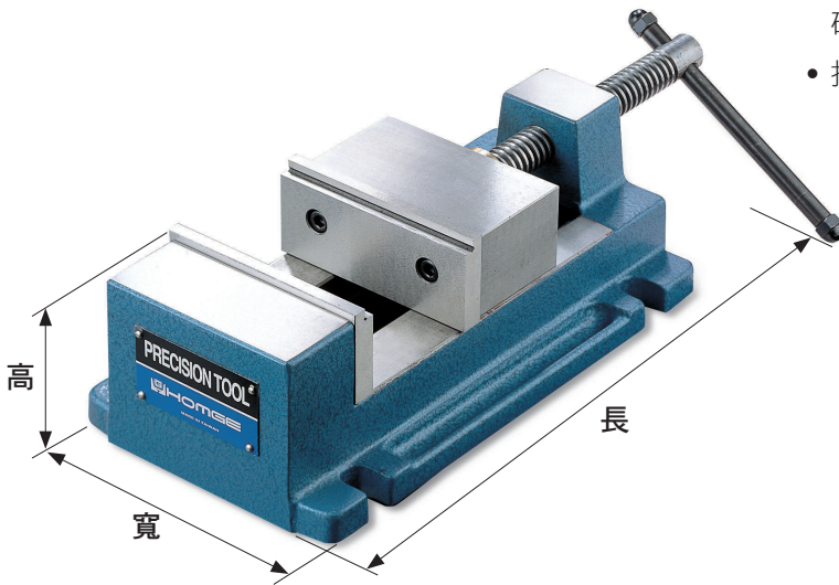
規格表 (材質: 高精度 FCD55 石墨鑄鐵)
