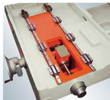
JHC-24H型下滑台之設計
